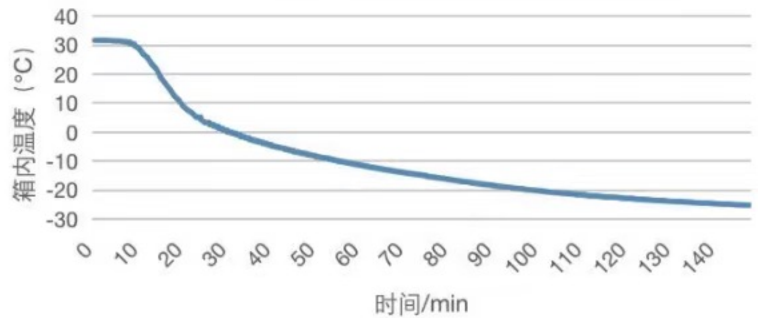
DW-25L400降温曲线图
