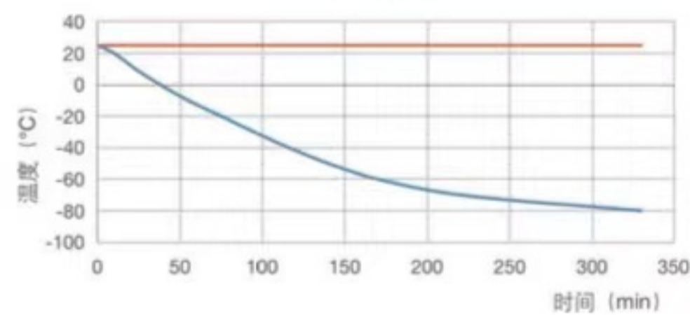
DW-86L707T降温曲线
