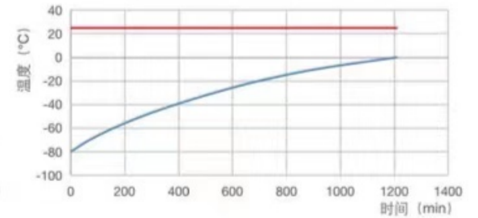
DW-86L707T回温曲线
